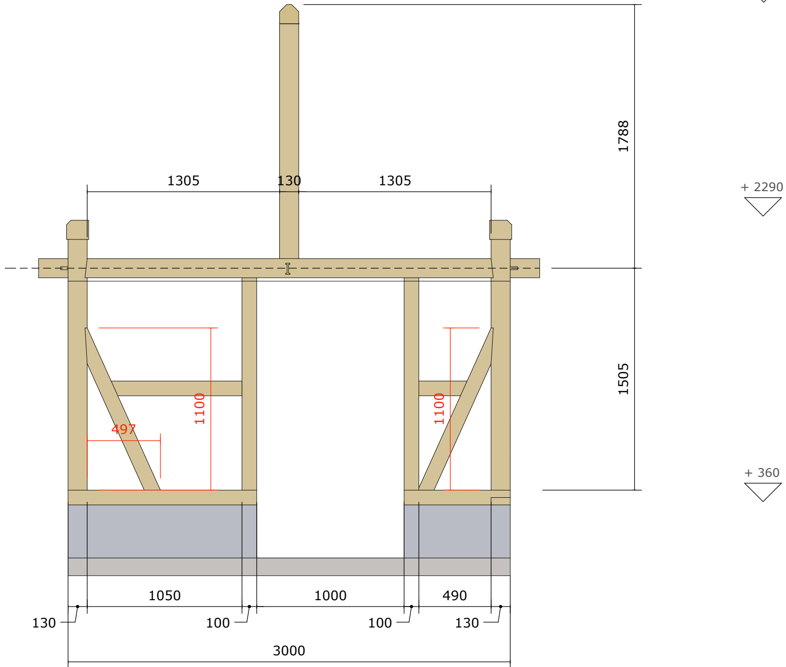
Aanzicht c straat 1:25
