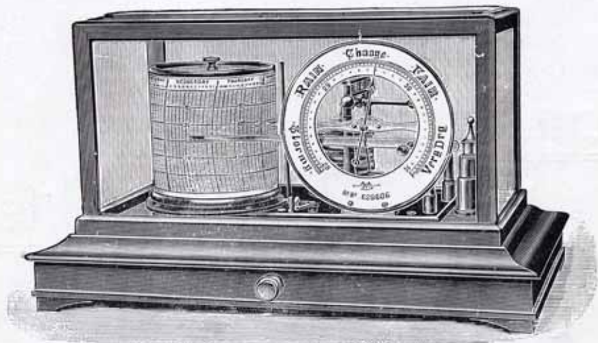
BAROMÈTRE ENREGISTREUR PERFECTIONNÉ MUNI DU CADRAN ANÉROÏDE
