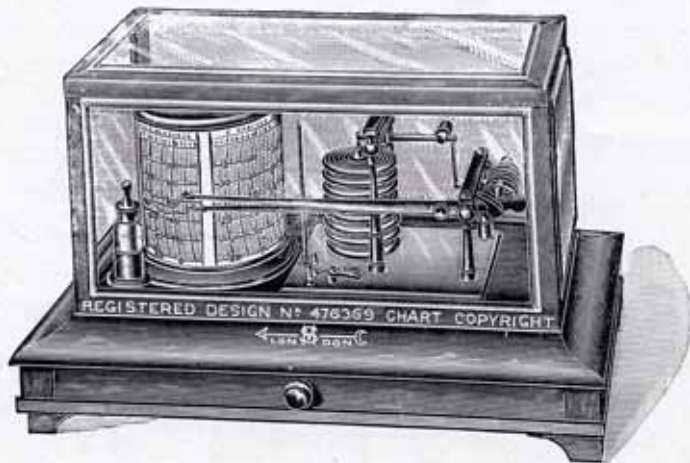
BAROMÈTRE ET THERMOMÈTRE ENREGISTREURS PERFECTIONNÉS
