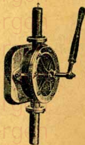
Pompes à palettes à effet double et quadruple, grand rendement. Se fabriquent en fonte et en bronze. Pour fonctionner à la machine ou à la main.
