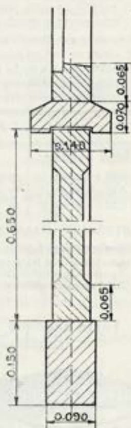
PLAN DE CLOISON VITRÉE AVEC COUPES
