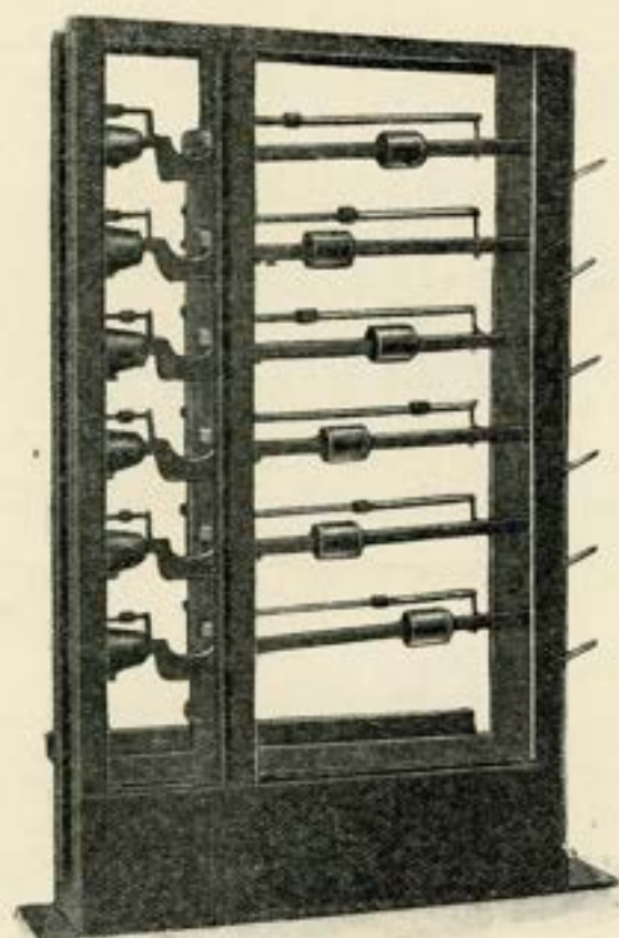
BASCULE à Romaines multiples
