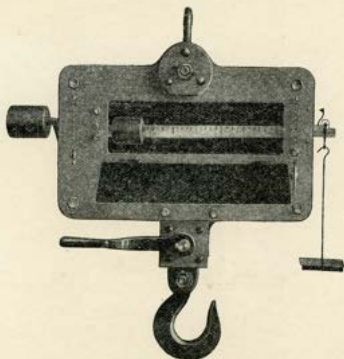
ROMAINE en l'air pour ponts roulants, grues, etc
