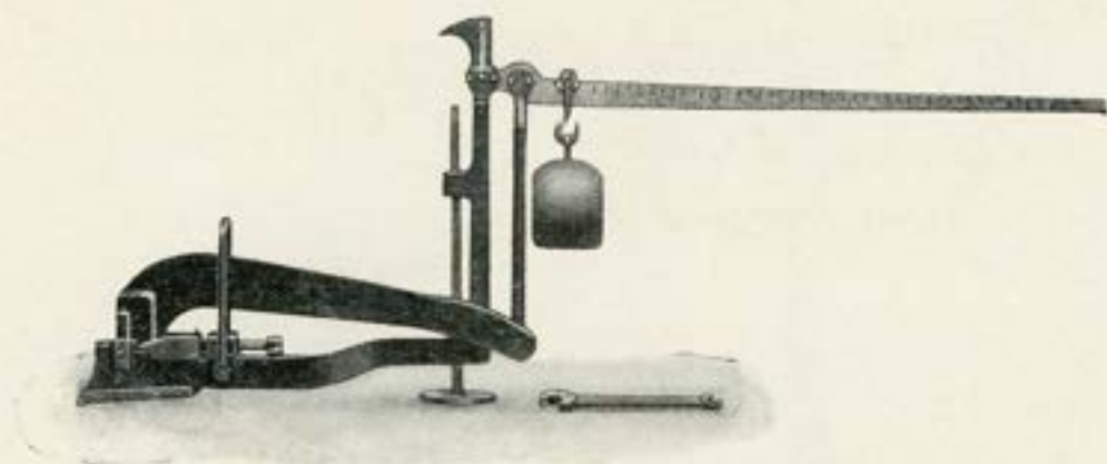
BALANCE-EHRARDT pour Locomotives
