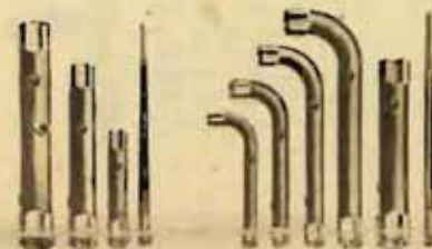
94. — CLEFS A DOUILLE, en acier, modèle renforcé. Droites 8-10 12-14 16-18 20-22 Prix 3,25 4.- 5,50 6,50 24-26 28-30 32-34 36-38 mm. 8,50 10,50 12.- 16,50 fr. coulées 12 16 20 26 30 mm. Prix 4,50 6,50 9.- 12.- 16 fr.
