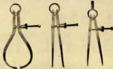
27 - 28 - 29. — COMPAS A RESSORT à serrage instantané par écrou fendu. Extr. long. 100 125 150 175 190 intér. à pointes / Prix 18.- 18,75 20,75 23,75 30 fr.
