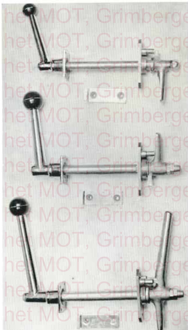
Verscheidene modellen van handgrepen Divers modèles de poignées
