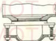
Raccord à collet pour tube plomb.
