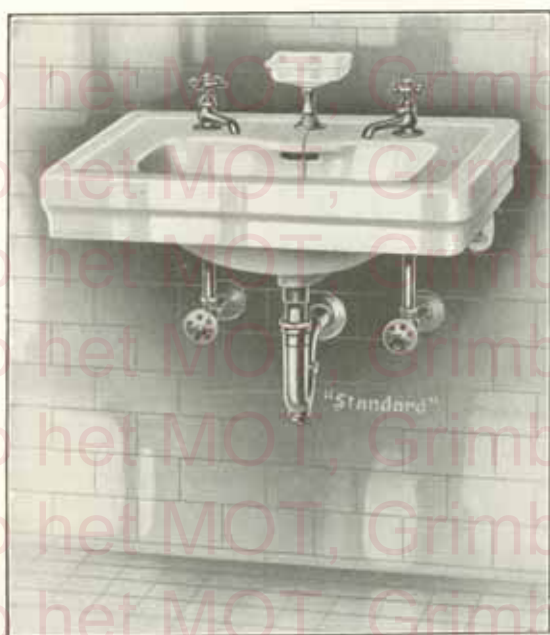
Lavabo sur consoles CRANSTON Porcelaine vitrifiée "Standard"
