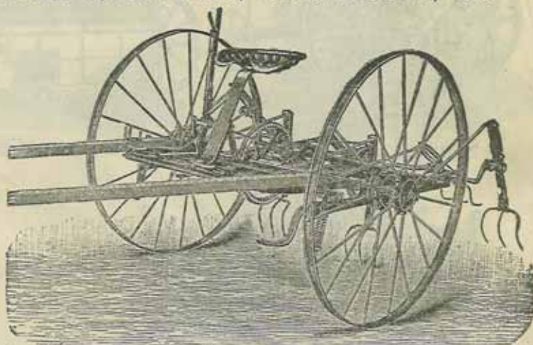
Faneuse à fourches.
