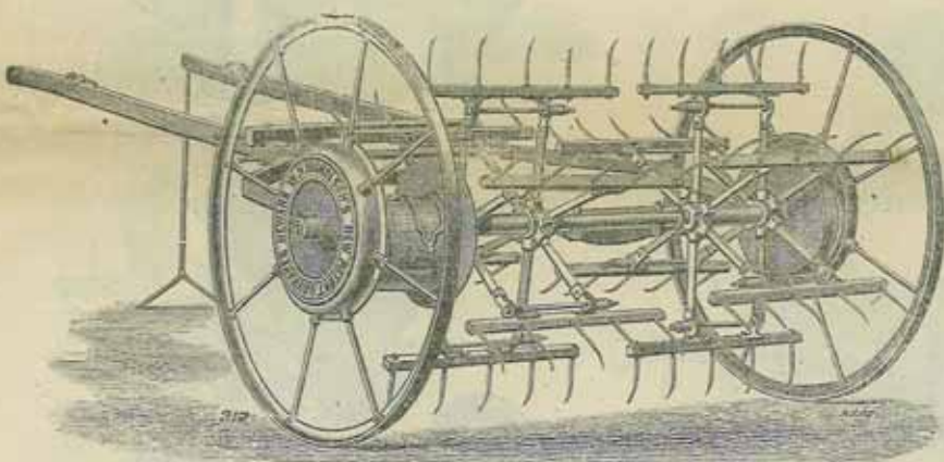
Faneuse "Rotative", à double action.
