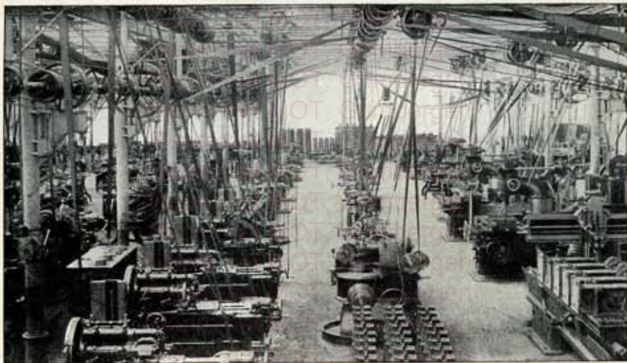
Vue intérieure des Ateliers. - Hall des Machines-Outils. - Section des Machines à tailler les engrenages
