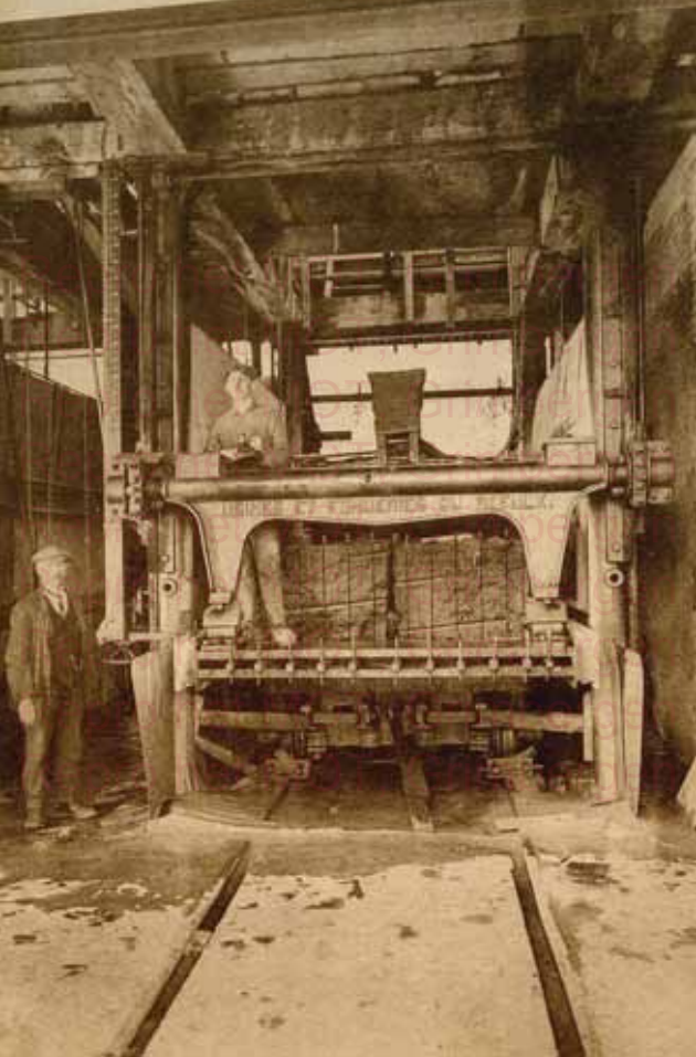
Vue d'un châssis à scier, Aanzicht van eene zaagmachien.
