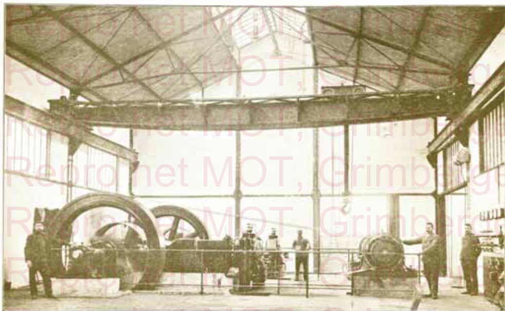
Distilleries Bal, à Merxhem. — Nouvelle centrale, salle des machines et pont roulant.
