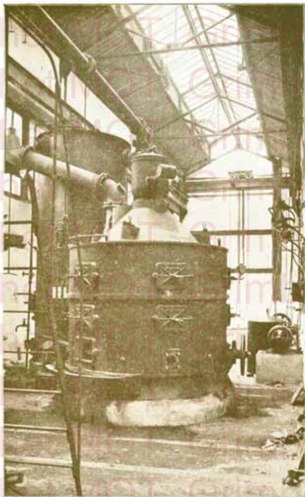
Distilleries Bal, à Merxem. Nouvelle centrale, salle des gazogènes.
