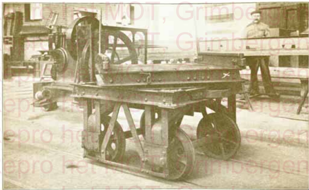
Wagonnets spéciaux pour magasins de fer, dépôts de poutrelles.
