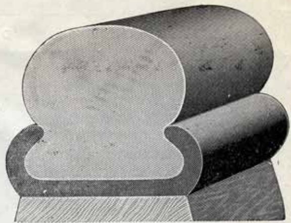
SECTION 51, Acier de 51 millimètres pour victorias, coupés, tonneaux, voitures à deux roues
