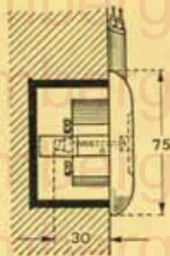
Interrupteur pour clef mobile. Entrée de fil cuirassé sur le mur
