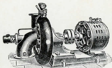
Pompe centrifuge à haut effet, brevetée accouplée directement à un moteur électrique.
