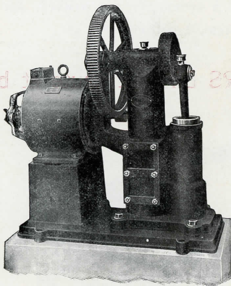
Pompe à piston Simplex à commande par moteur électrique.
