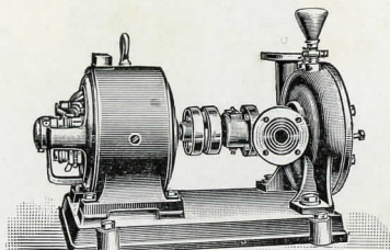
Pompe à développantes électrique.
