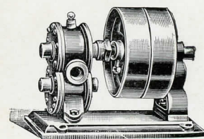
Pompe rotative fig. 388
