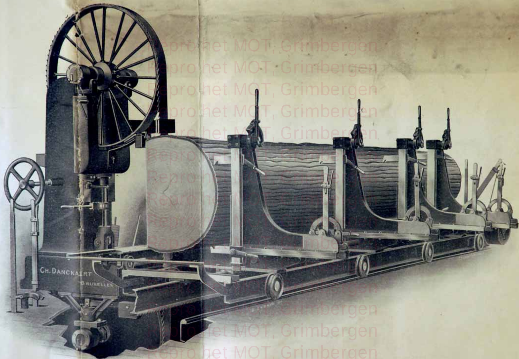
SCIE A RUBANS POUR LE DEBIT DES BOIS EN GRUMES.
