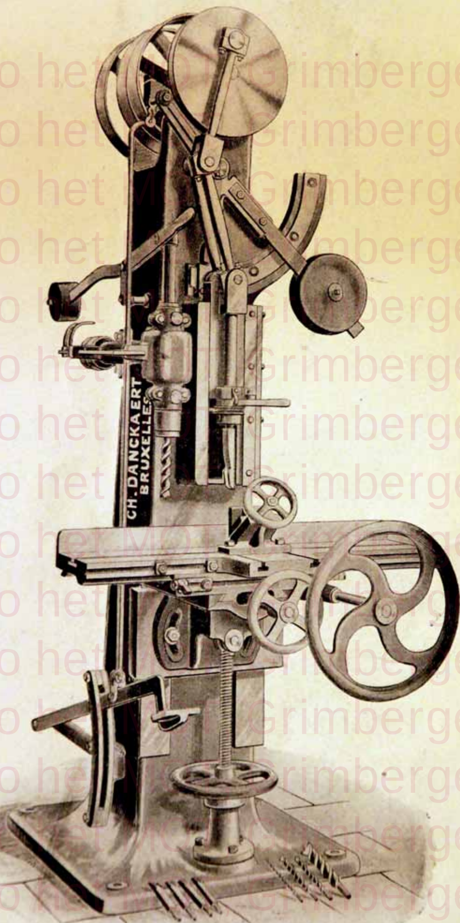
MORTAISEUSE VERTICALE.
