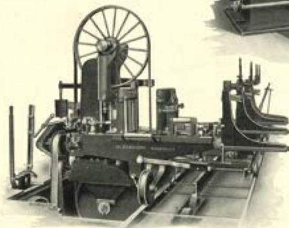
WALSEN LINTZAAGMACHINE Zaagwielen : 1.100 en 1.250 m.
