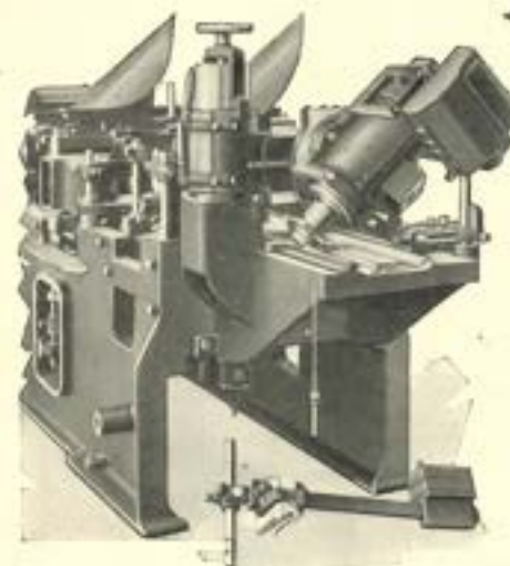
DERDE VERTIKALE BEITELAS welke op iedere vierzijdige van 275 × 125 en 375 × 125 kan worden aangebracht.
