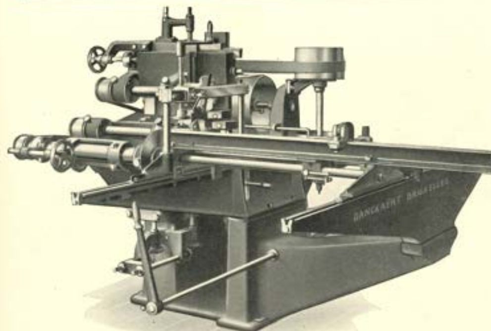
PENNENBANK VOOR PENNEN TOT 150 M/M LANG.
