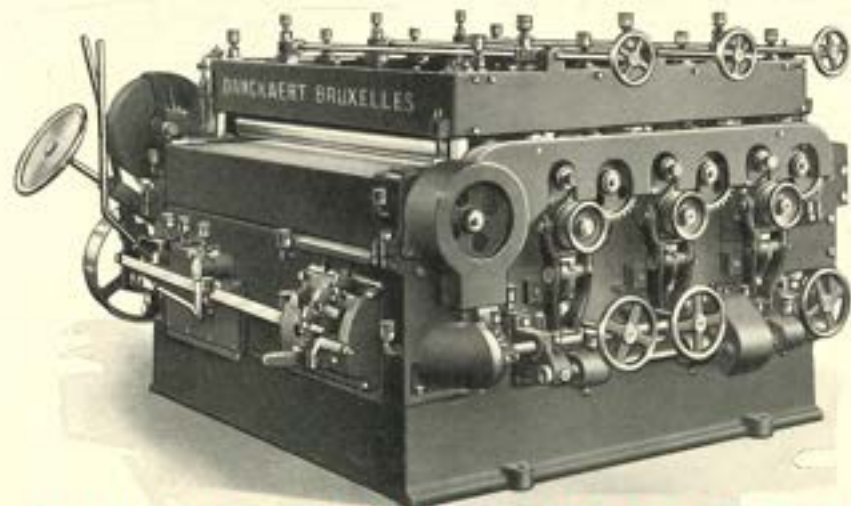
SCHUURMACHINE MET 3 CYLINDERS EN AANVOER DOOR WALSEN Voor hout tot 1010 \times 200 m/m, 1270 \times 200 m/m, 1670 \times 200 mm.
