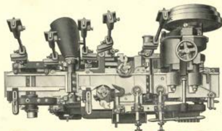
VIERZIJDIGE LIJSTENSCHAAFMACHINE MET VIER OF VIJF ASSEN. — VOOR HOUT TOT 180 × 80. Drie aanvoersnelheden.
