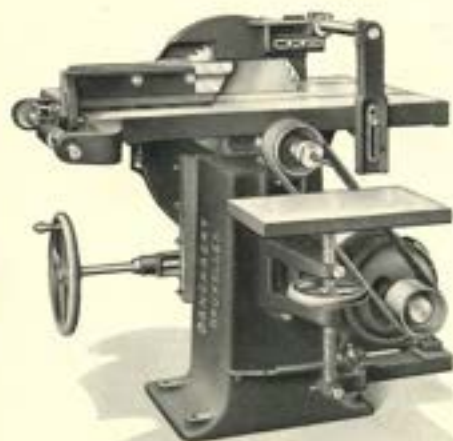
Machine met eenvoudig booreapparaat.
