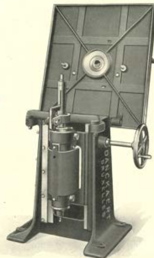
DE TAFEL OPGEKLAPT en de machine voorzien van bokfraisapparaat.
