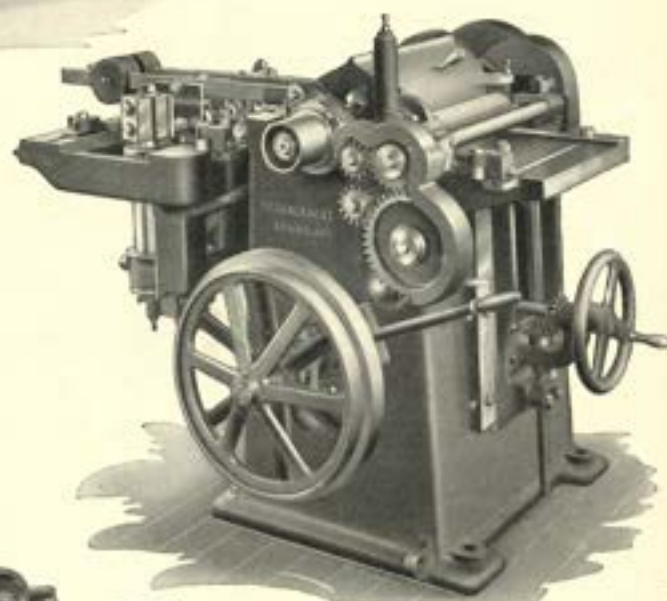
DRIEZIJDIGE SCHAAPMACHINE voor hout tot 400 \times 180 en voor 700 \times 220 .
