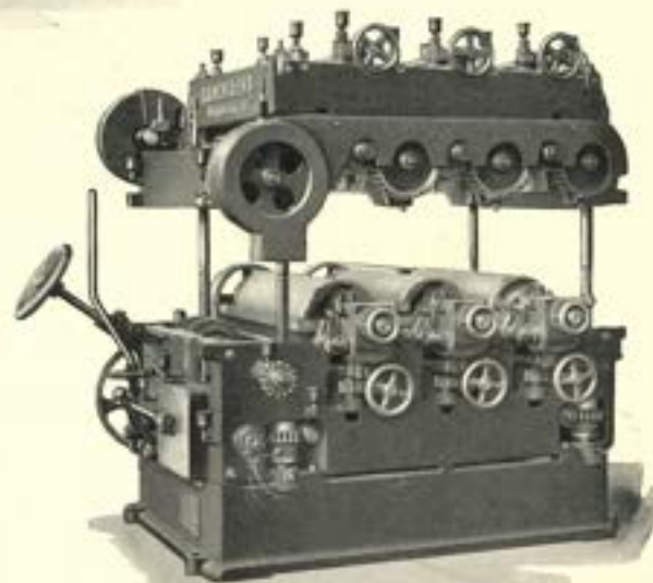
Het bovengedeelte is automatisch omhoog gebracht teneinde gemakkelijk bij de schuurcilinders te kunnen komen.
