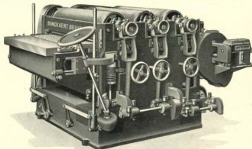
SCHUURMACHINE MET DRIE CYLINDERS AANVOER DOOR TAPEL ZONDER EINDE Voor hout tot : 1.014 \times 0.15 m. en 1270 \times 0.15 m.
