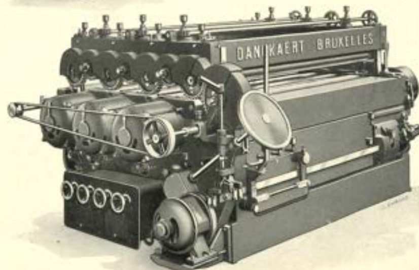
SCHUURMACHINE MET 3 CYLINDERS EN AANVOER DOOR WALSEN MET INGEBOUWDE MOTOREN.
