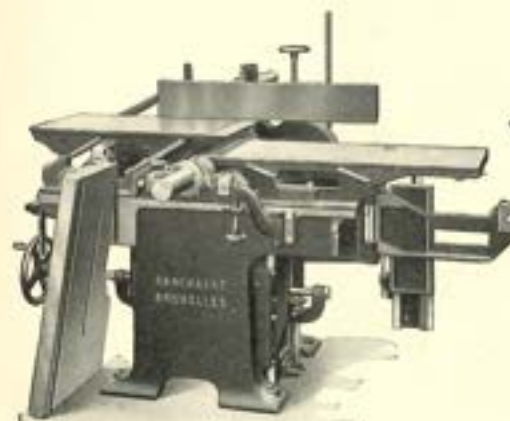
MACHINE OESTELD VOOR VANDIKTESCHAVEN
