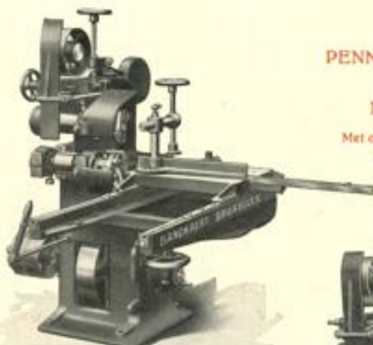
SPECIAAL MODEL VOOR STOELFABRIEKEN MET OF ZONDER AFKORTZAAG
