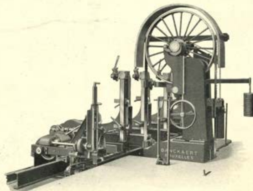
BOOMLINTZAAGMACHINE MET AUTOMATISCHE DIKTEINSTELLING
