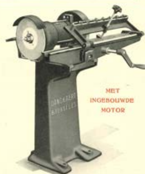
SLIIPMACHINE VOOR RECHTE- EN PROFIELBEITELS
