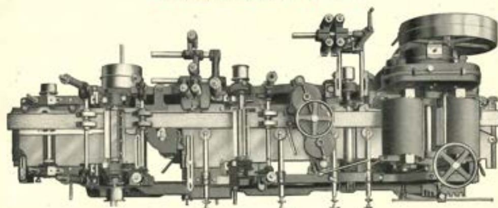
Bovenaanzicht.
