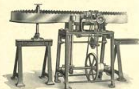
MACHINE VOOR HET OP BREEDTE BRENGEN VAN GESTUIKTE TANDEN
