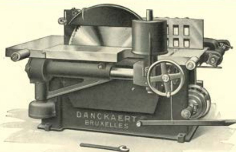
CIRKELZAAGMACHINE voor zaagbladen tot 900 m/m met automatische aanvoer.
