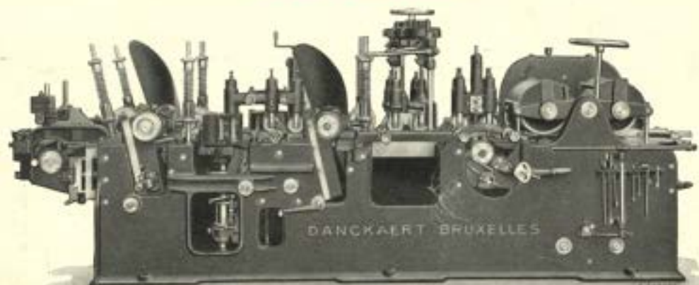
VIERZIJDIGE SCHAAFMACHINE MET 6 ASSEN EN VASTE MESSEN voor hout tot 275 \times 125 en 375 \times 125 . Kan ook worden geleverd zonder kraalblok.
