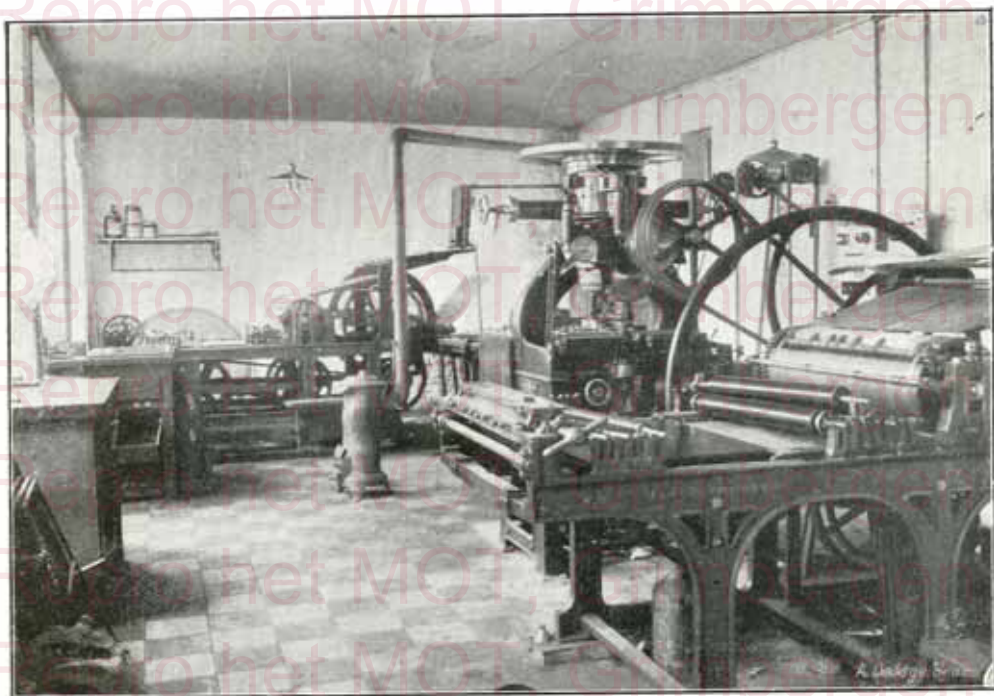
ATELIER DE TIMBROGRAVURE
