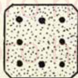
Fig. 19 Disposition des armatures dans le pieu d'angle.
