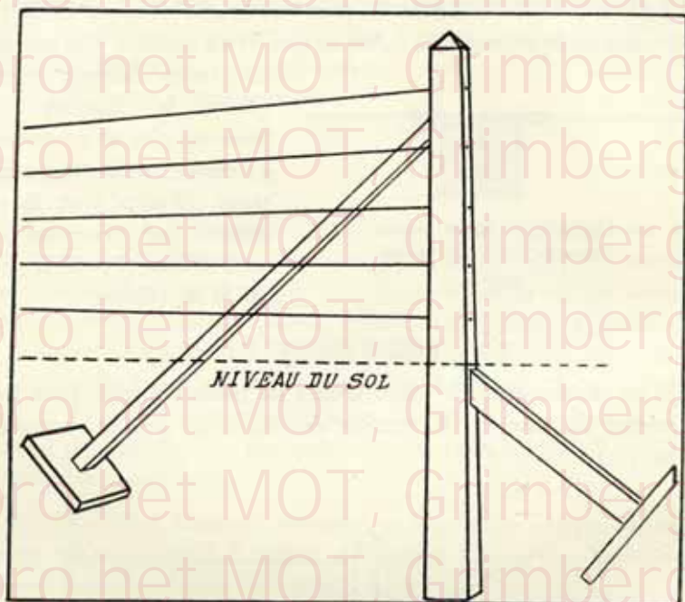
Fig. 18. — Modèle du pieu renforcé avec étais.
