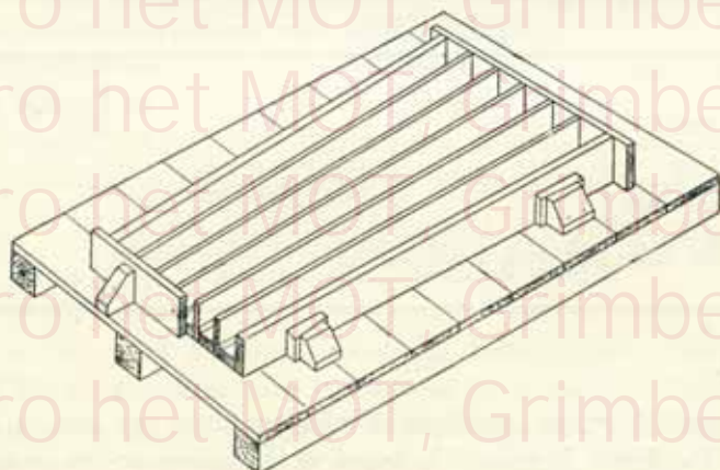
Fig. 2. — Moule pour pieu à section réduite à la tête.
