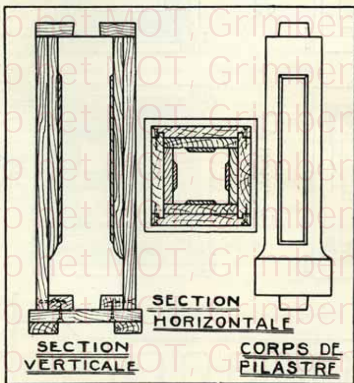
Fig. 28. — Corps de pilastre.
