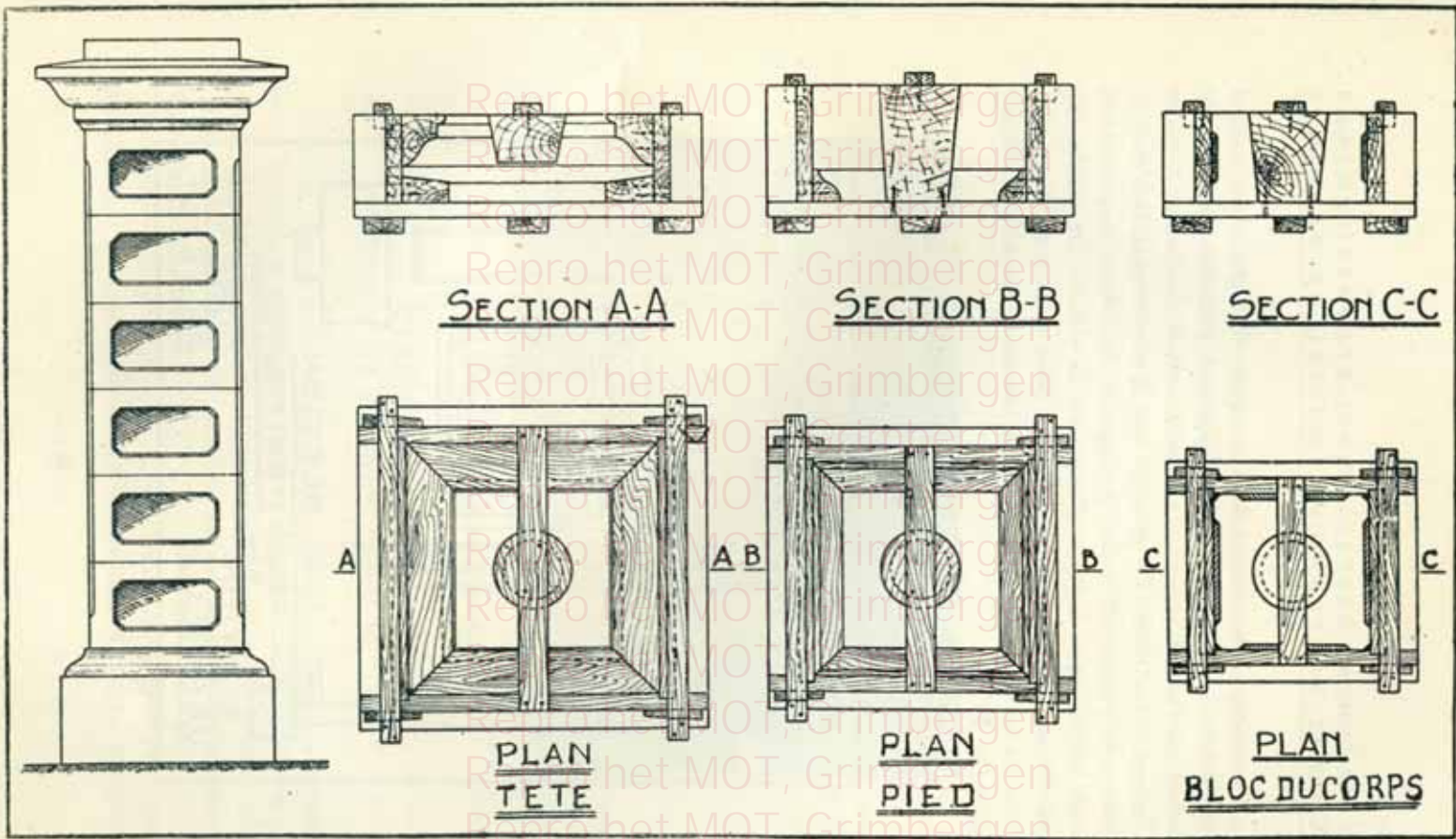
Fig. 27. — Type de pilastre pour grille.
