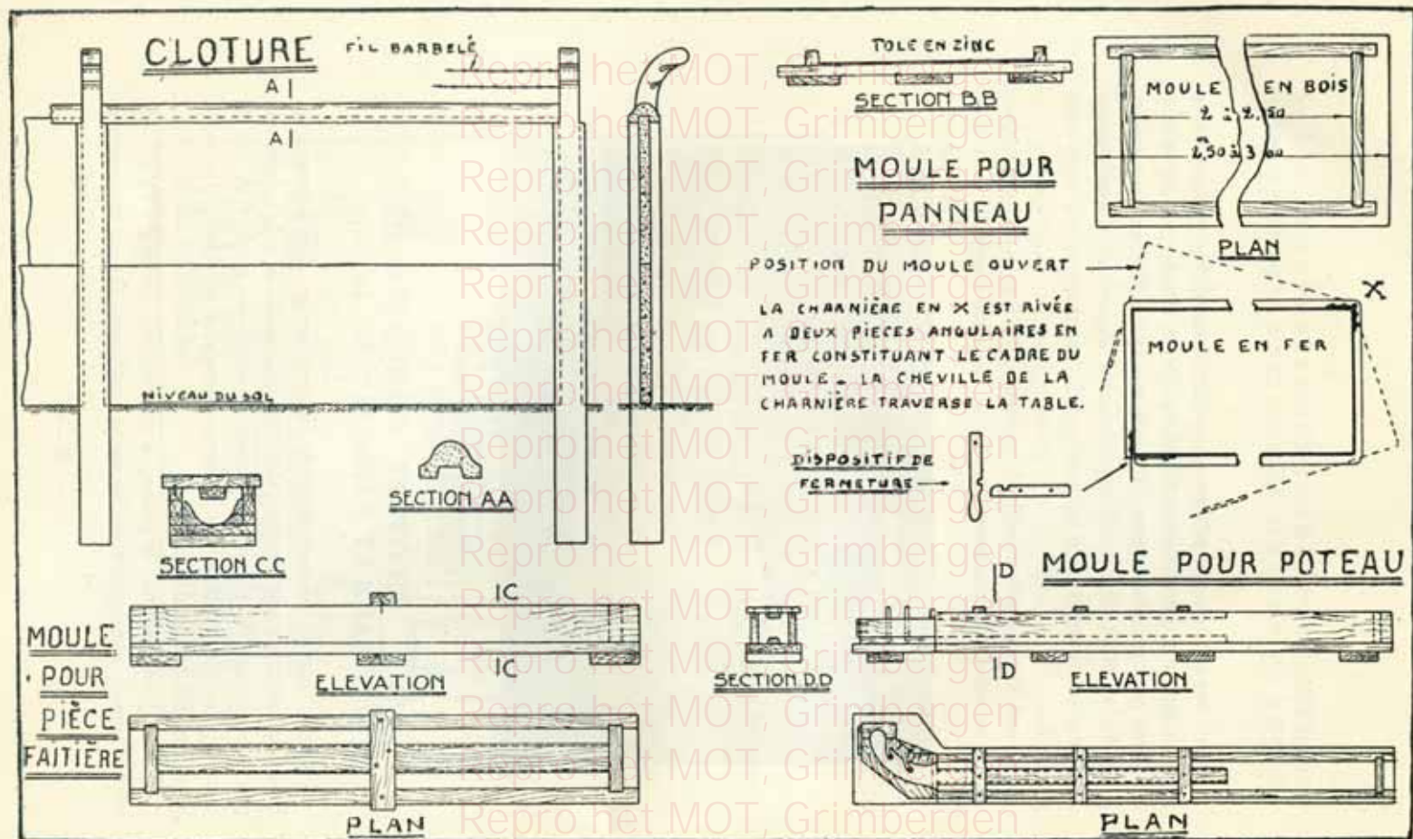
Fig. 30. — Clôture composée de poteaux et panneaux en béton.
