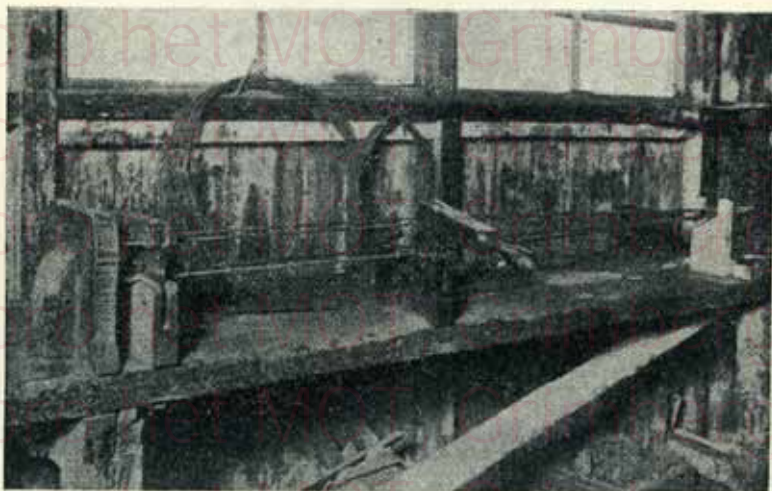
Fig. 9. — Dispositif d'ensemble permettant de confectionner aisément les armatures métalliques pour pieux.
