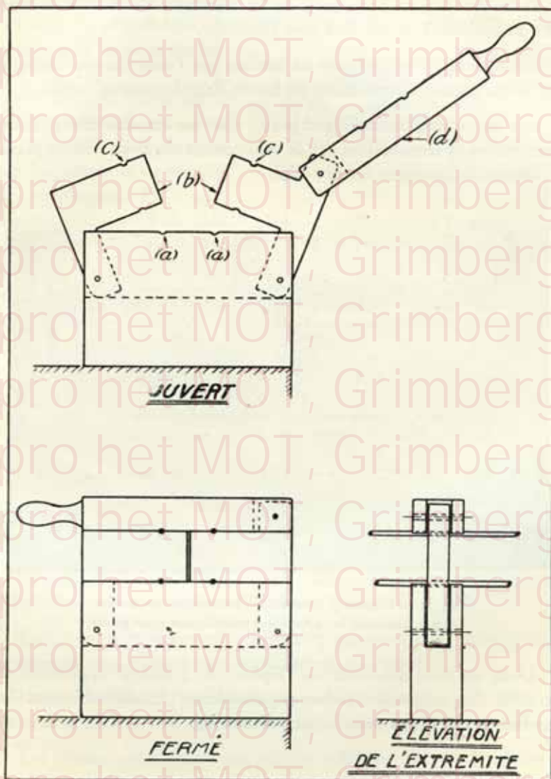
Fig. 8. — Détails du dispositif permettant d'immobiliser les barres pendant la confection des armatures.
