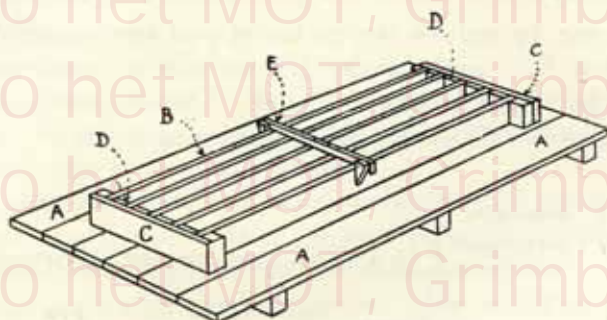
Fig. 1. — Moule pour pieux à section constante.
