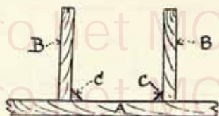
Fig. 4. — Moule pour pieu garni de réglettes en bois C, moulant les pans coupés inférieurs.
