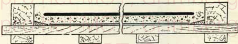
Fig. 32. — Coupe dans un moule pour panneau.
