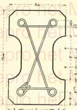
Fig. 19. — Section de la poutre de toiture dans la partie en double T.
