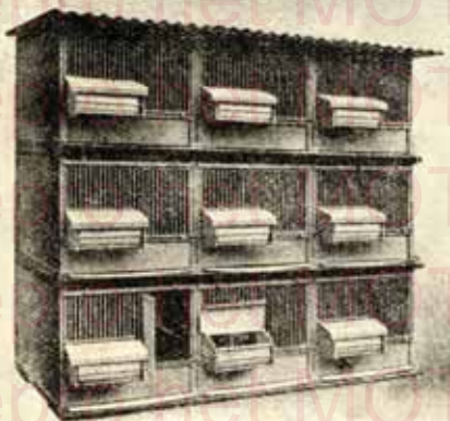
Fig. 34. — Clapier en bois avec toiture en fibro-ciment.
