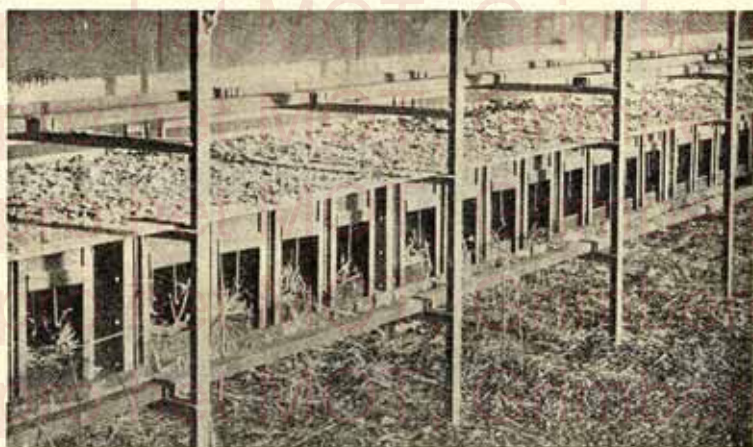
Fig. 16. — Nids-trappes et planches à déjections. Application des produits en fibro-ciment. Cliché mis obligeamment à notre disposition par la S. A. Eternit.
