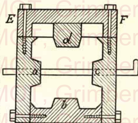
Fig. 18. — Coupe dans le moule pour pieu.
