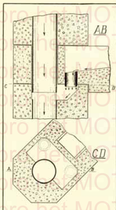
Fig. 25. — Coupe montrant le dispositif pour l'écoulement.
