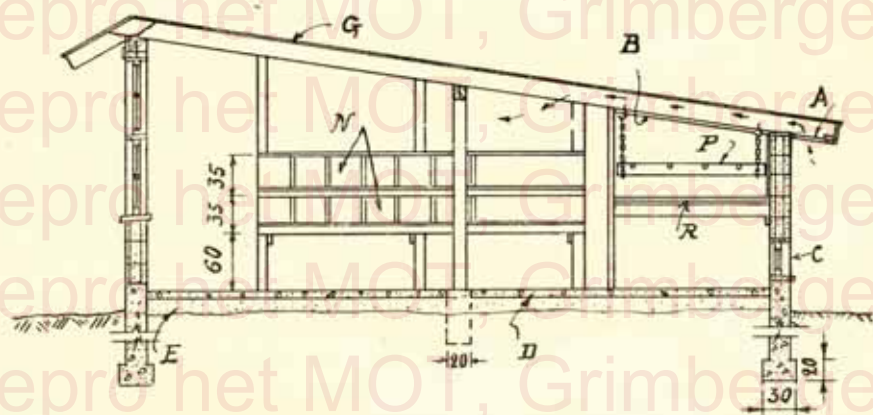
Fig. 7. — Section transversale.
