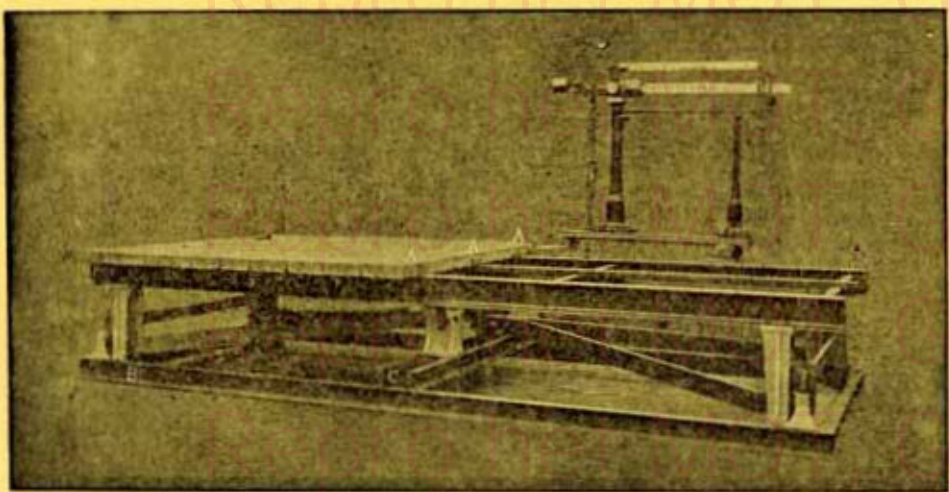
Pont à peser les chariots, assise en acier, (B) supprimant l'emploi des pierres de fondation, doguets, etc,
