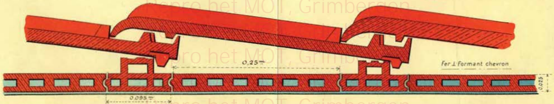
Coupe dans l'axe d'une tuile posée
