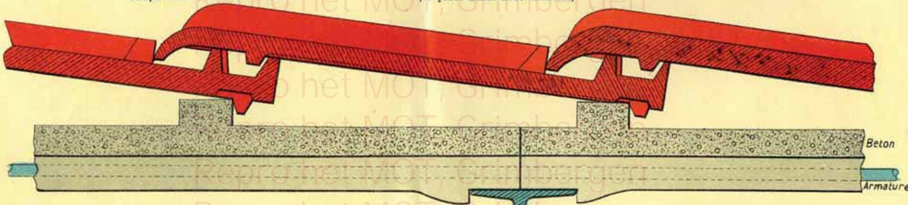
Coupe dans l'axe d'une tuile
