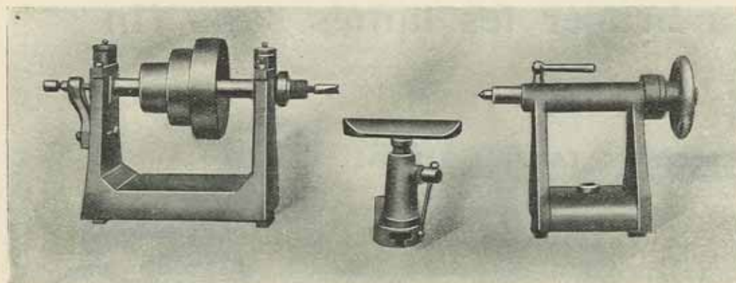
JB. Garniture du tour (Fort modèle)
