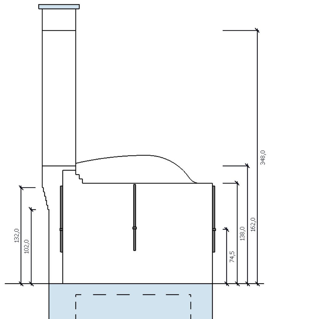
zijaanzicht NT
