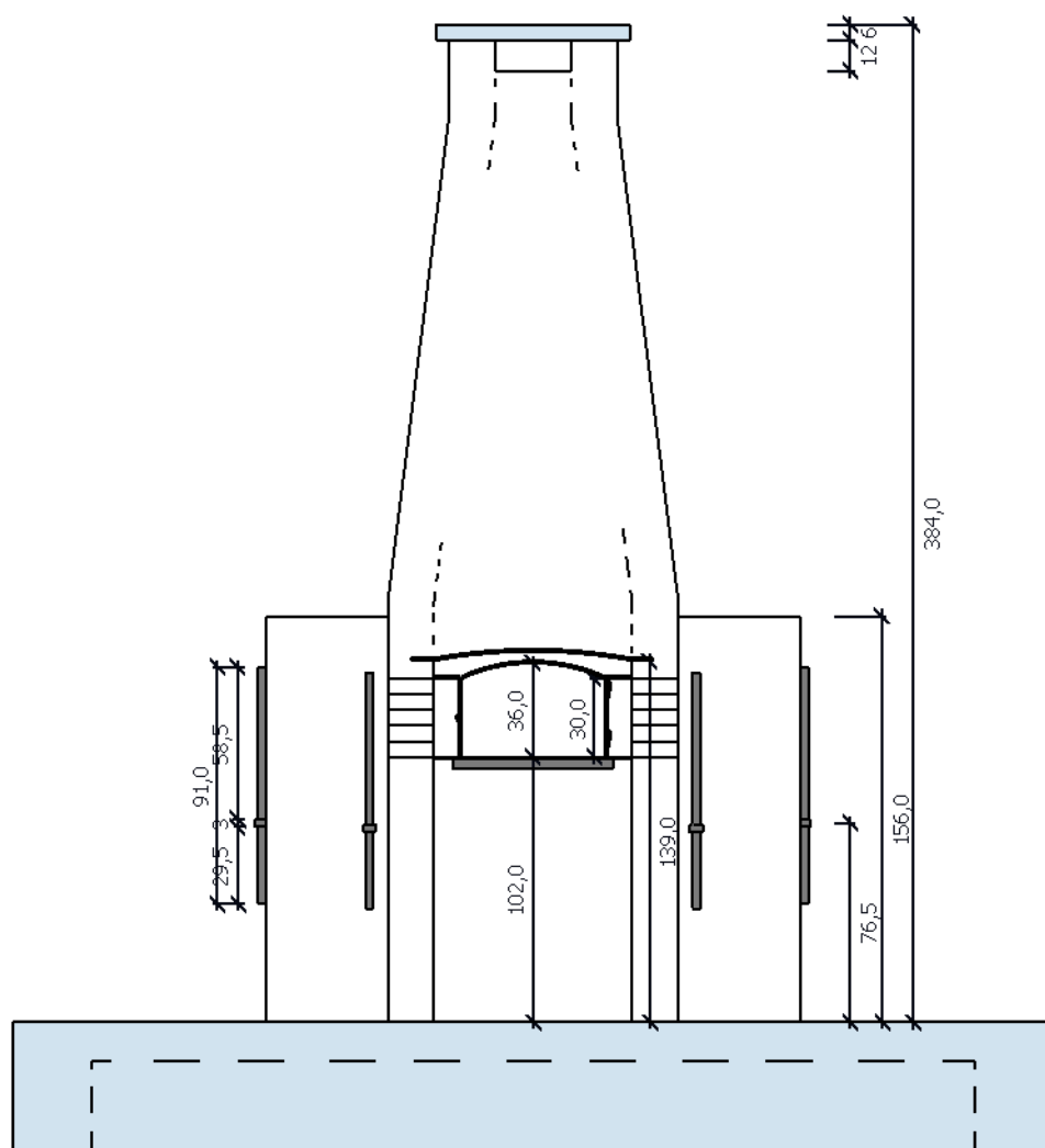
vooraanzicht NT
