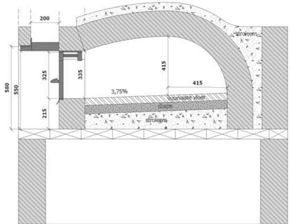
snede A
