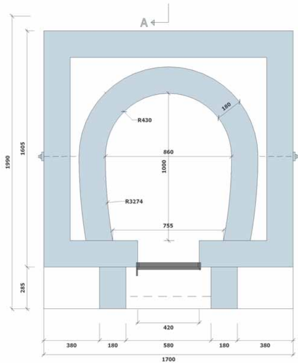
grondplan
